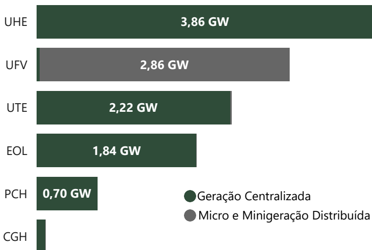
Capacidade Instalada Acumulada por Fonte
